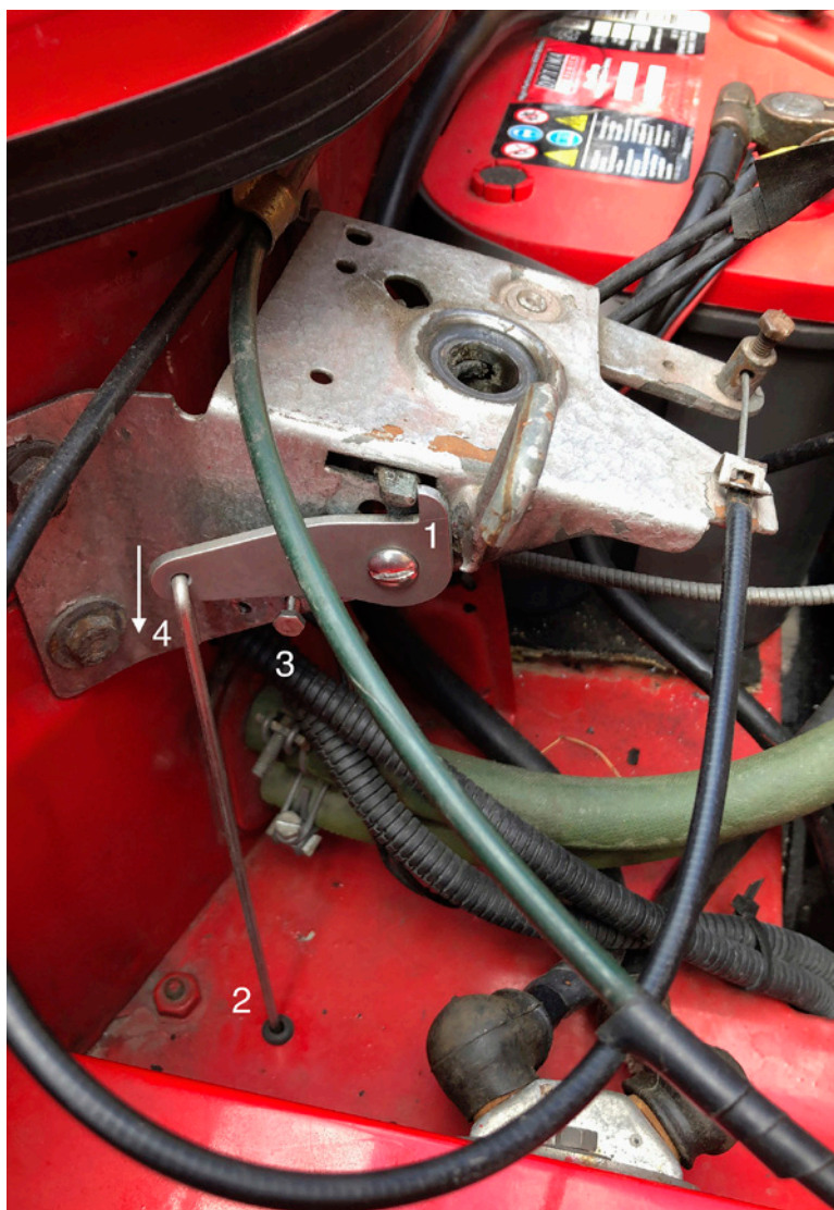
Alla delar som följer med. Det bifogas även en stoppskruv som förhindrar "spaken/kroken" att passera spärren när du drar i länkaget.
